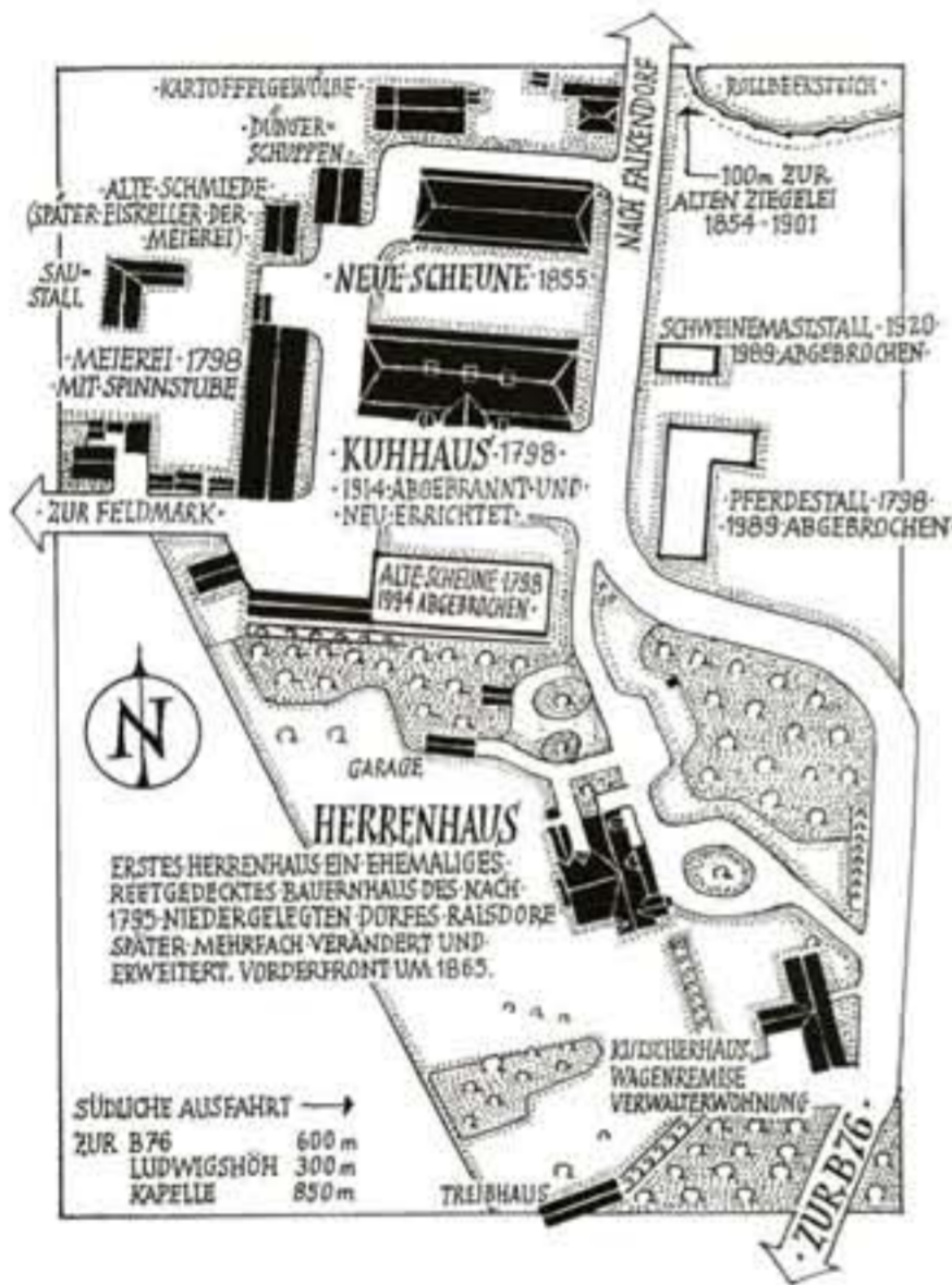
Plan der Hofanlage Gut Sophienhof
