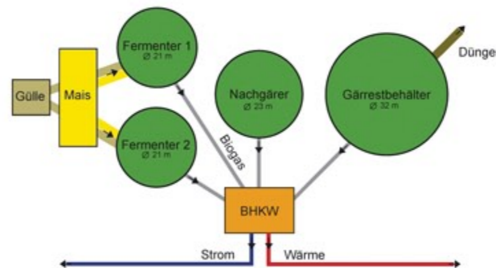
Schema einer Biogasanlage mit zwei Fermentern
